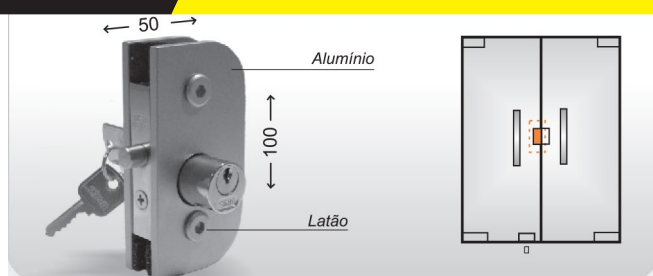
CÓD 1520 Fechadura de centro com 2 cilindros
