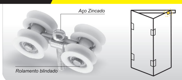
CÓD 1150 Roldana quadrupla para trilho 1030
