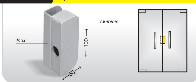
CÓD 1504 P Contra fechadura de pressão para 1520 P
