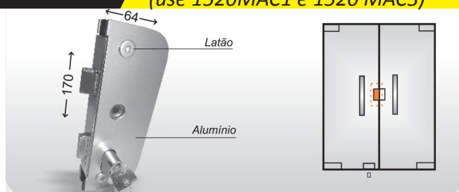
CÓD 1520 MC Fechadura de centro com 2 cilindros sem maçaneta (use 1520MAC1 e 1520 MAC3)
