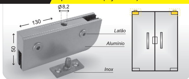
CÓD 1101 Dobradiça pivotante superior com pivot 1009 (aço inox)
