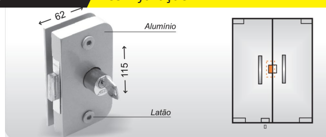
CÓD 1520 X Fechadura para porta de abrir com furação
