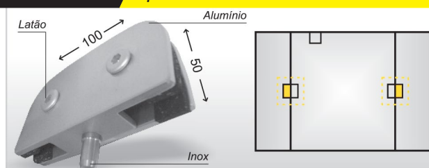
CÓD 1130 Dobradiça com pino (Aço inox) para basculante 50x100mm
