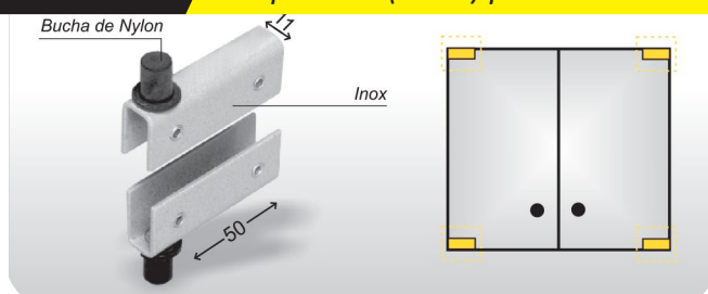
CÓD 1141 P Conjunto de dobradiças pivotantes de pressão (6mm) para rack
