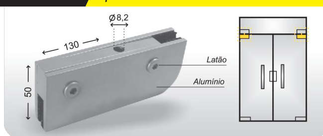
CÓD 1101 A Dobradiça pivotante superior para 1203 e 1209
