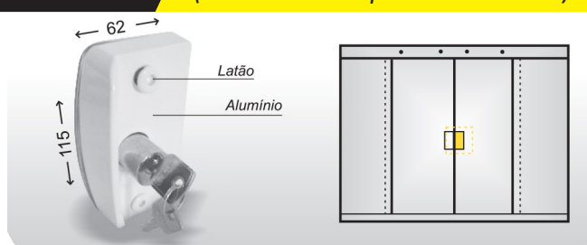
CÓD 1510 XA Fechadura para janela de correr (sem cilindro e puxador externo)
