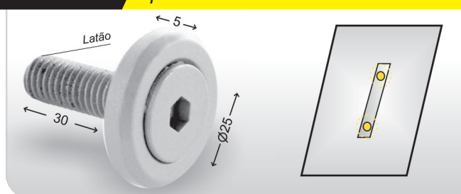
CÓD 1010 Botão de acabamento avulso para puxador 1676 S
