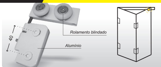
CÓD 1125 SF Roldana para box sanfonado
