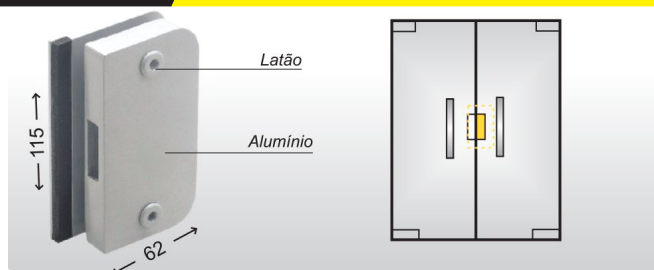
CÓD 1504 AX Contra fechadura V/V com aba para 1520 X
