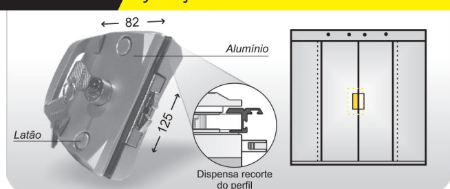
CÓD 1510 BX Fechadura para porta de correr furação Blindex 3530
