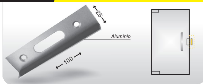
CÓD 1504 B Batedeira em alvenaria para 1520
