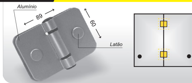
CÓD 1137 Dobradiça dupla para janela
