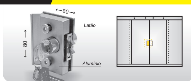
CÓD 1510 M Mini fechadura para porta de correr
