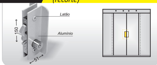
CÓD 1510 Fechadura bico-de-papagaio com pino trava para porta de correr (recorte)
