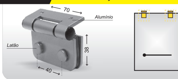
CÓD 1132 Dobradiça pra maxim-ar V/A 40mm entre furos
