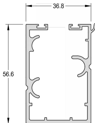
Trilho superior
