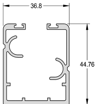
Trilho inferior
