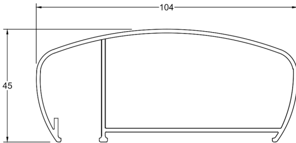
GR-001 Corrimão
