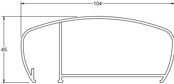
GR-001 Corrimão
