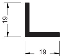
CT-007 Cantoneira de Arremate
