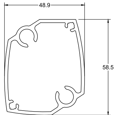
GR-008 Chumbador
