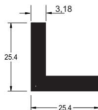
ALM0656 Cantoneira reforçada
