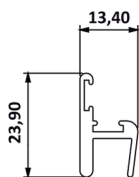
CADEIRINHA
