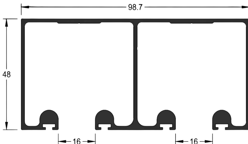
BX001 - TRILHO SUP. QUÁDRUPLO
