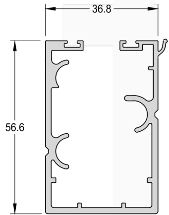
Trilho superior
